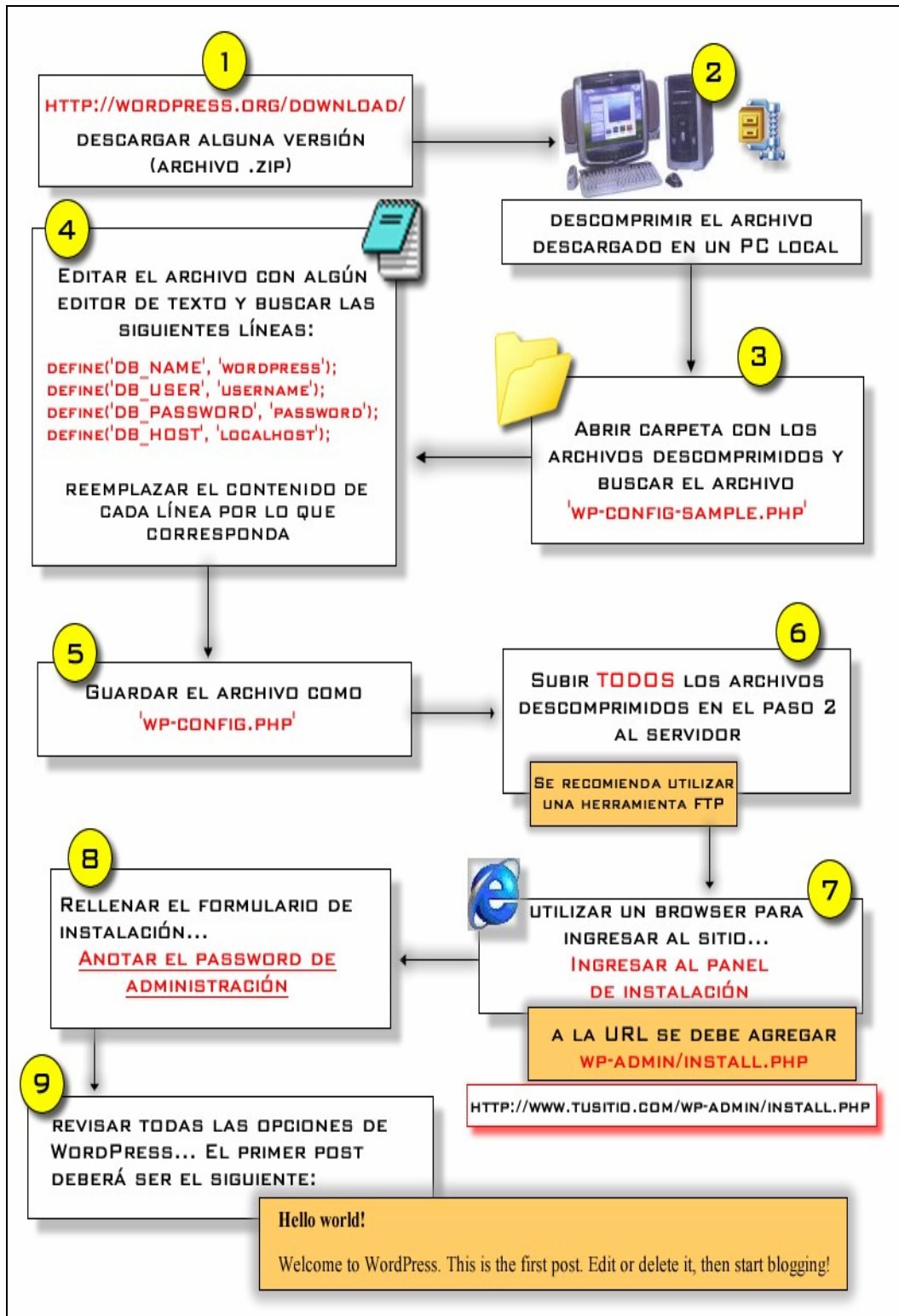
Figura 6 Instalación de WordPress
